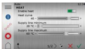
Fig. 4: Réglages du chauffage
